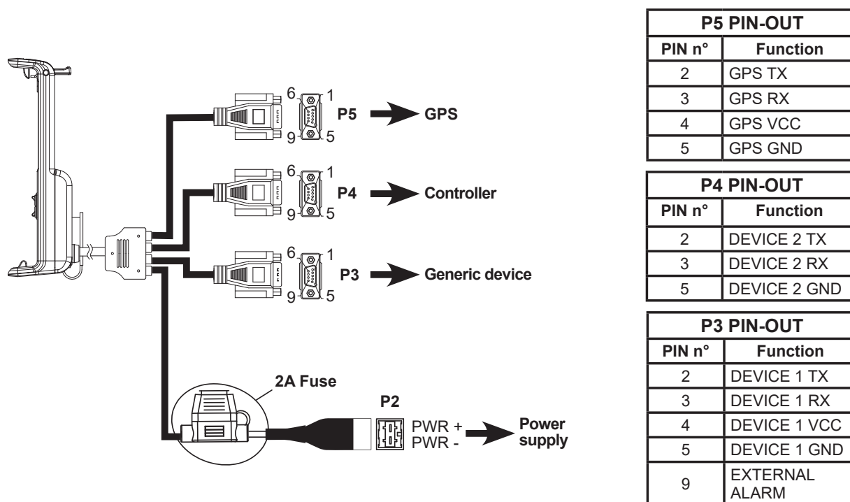
Figura 1.2 - Schema di collegamento elettrico
