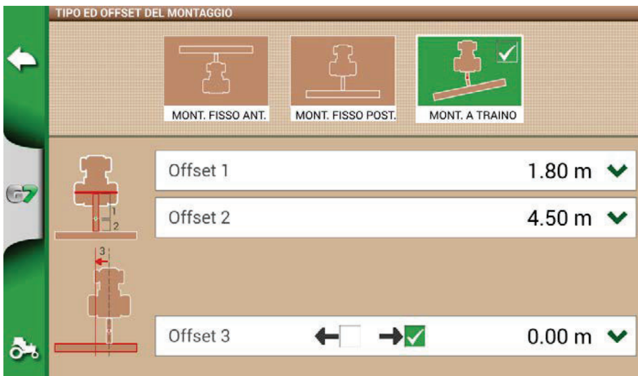
Figura 2.1.6.f - Attrezzo con montaggio posteriore snodato
