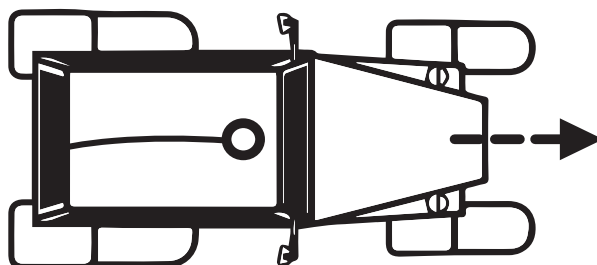
Figura 1.3.5 - Come installare l'antenna - Orientamento
