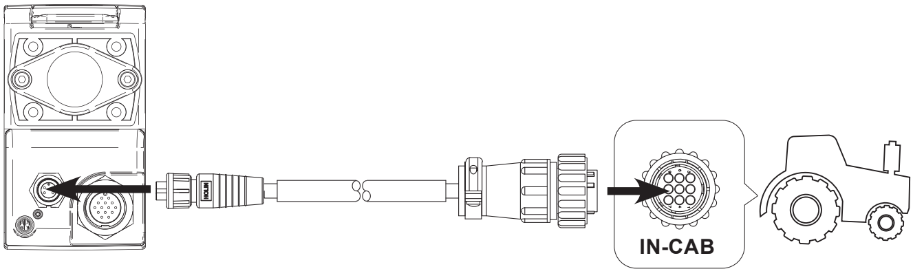
Figura 1.2b - Schema di collegamento ISOBUS In-Cab
