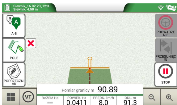
Mapowanie pól
