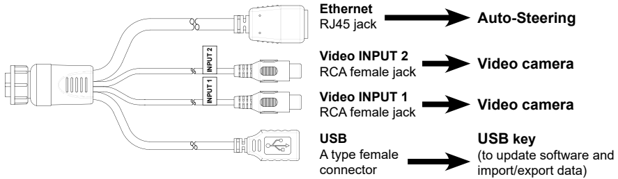
Figura 5.1.a - Cavo USB +Video in + Eth + 2 camere
