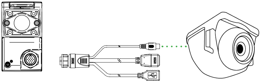
Figura 6.4.2 - Collegamento di una videocamera a G12 Panorama
