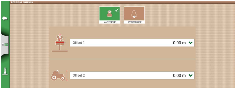
Figura 2.4.2 - Pagina di configurazione della posizione dell’antenna
