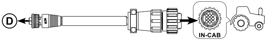
Figura 1.2.d - Schema di collegamento ISOBUS In-Cab
