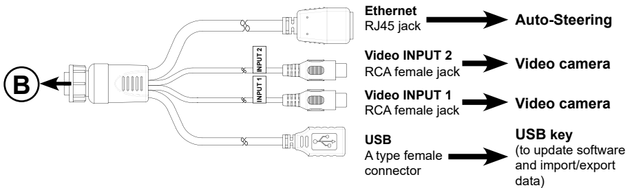
Figura 1.2.c - Schema di collegamento ISOBUS In-Cab
