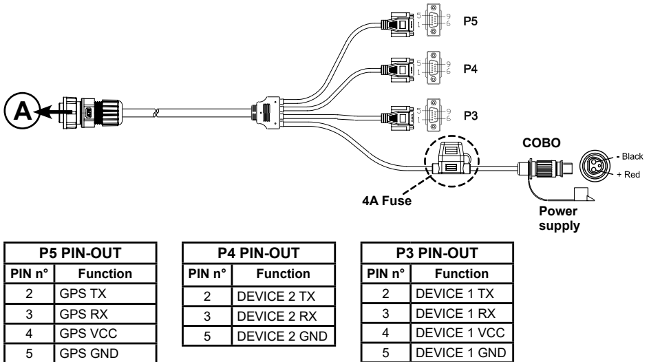
Figura 1.2.b - Schema di collegamento elettrico
