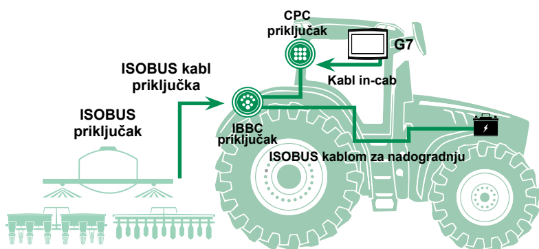
Vozila koja nemaju ISOBUS
