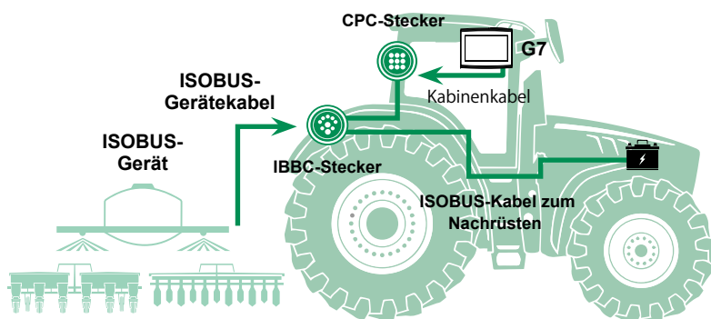
Nicht-ISOBUS-Fahrzeuge
