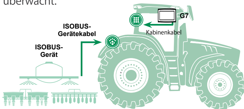
ISOBUS-fähige Fahrzeuge
